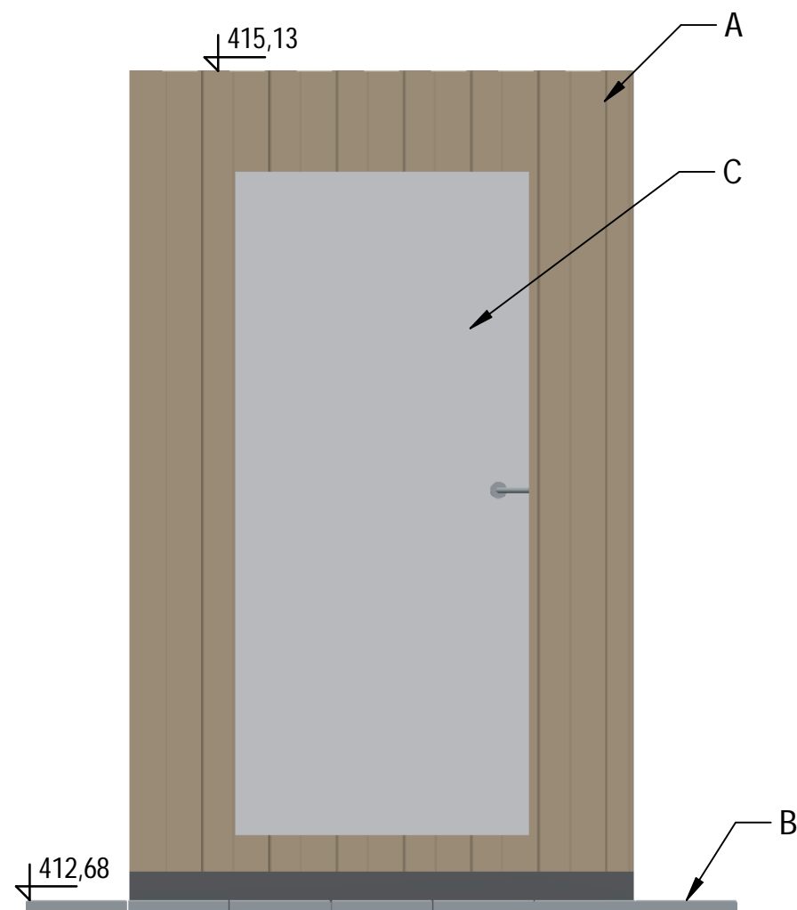
POHLED VÝCHODNÍ
