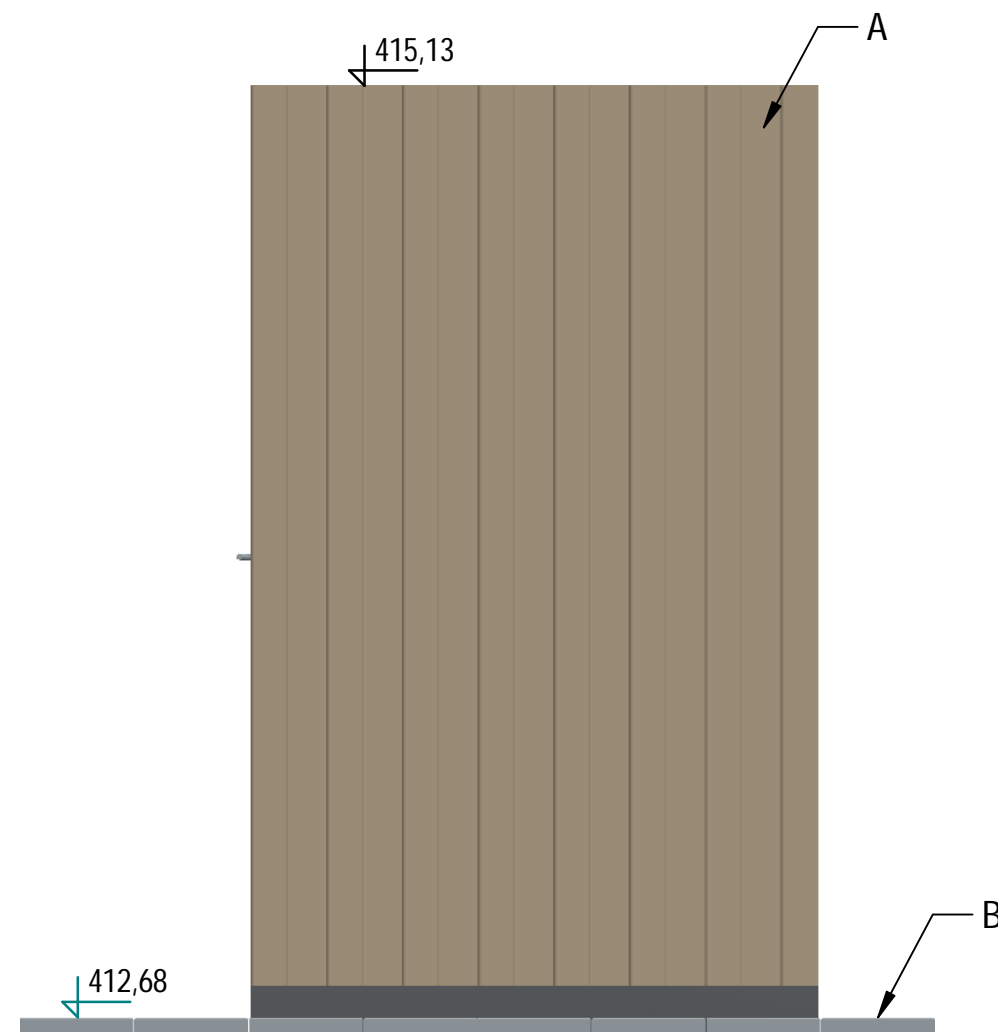
POHLED SEVERNÍ
